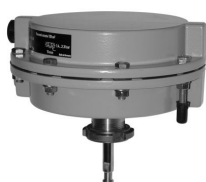
Fig. 4: Type 3271-5, 120 cm 2
