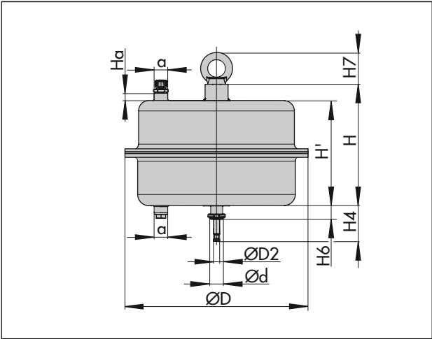
Bild 3: Typ 3271 mit 1000 cm² Antriebsfläche
