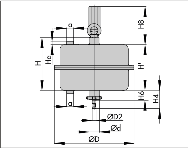
Bild 4: Antriebsfläche 1000 cm², mit einstellbarer Hubbegrenzung
