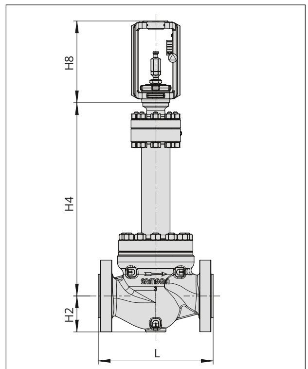
Bild 8: Ventil Typ 251GR mit Balgteil
