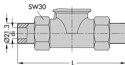
Регулирующий клапан с концами под пайку
