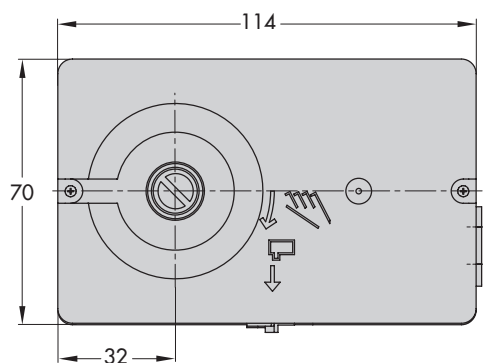
Тип 3222 N/5857 Тип 3222 N/5757-3 Тип 3222 N/5757-7
