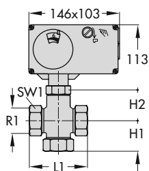
Typ 3226/5724-8: DN 15 bis 50 Typ 3226/5725-8: DN 15 bis 50
