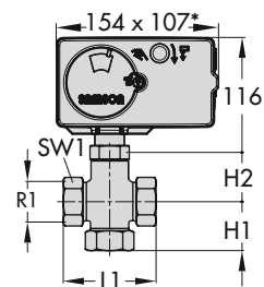
Typ 3226/5827: DN 15 bis 50 * Maße für Antriebe mit doppelter Stellgeschwindigkeit: 154 x 140
