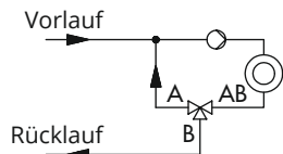
Bild 4: Einbaubeispiele
