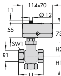
Typ 3226/5857: DN 15 bis 25 Typ 3226/5757-7: DN 15 bis 25
