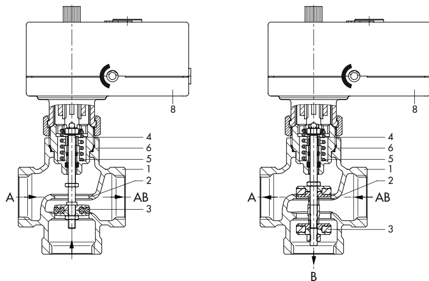
Bild 3: Wirkungsweise Typ 3226/5857 links: Mischventil, rechts: Verteilventil
