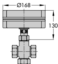
Typ 3226/2780-1: DN 15 bis 50
