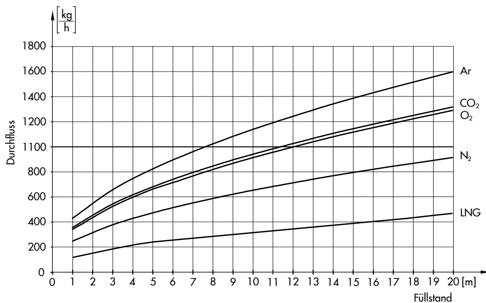
Bild 6: Massendurchfluss in Abhängigkeit von der Flüssigkeitssäule im Kryobehälter
