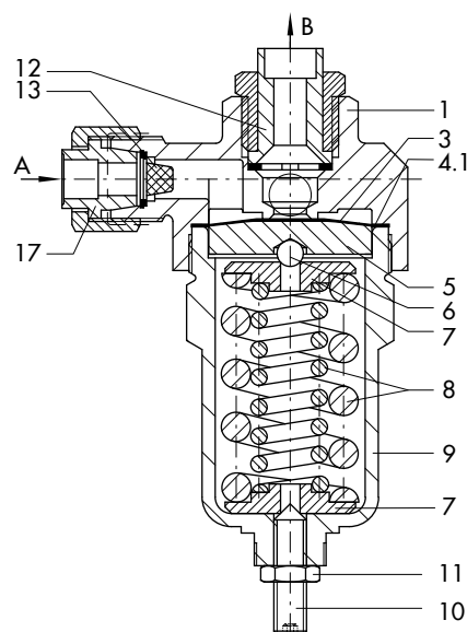
Bild 4: Überströmventil Typ 2357-2 (PN 50)
