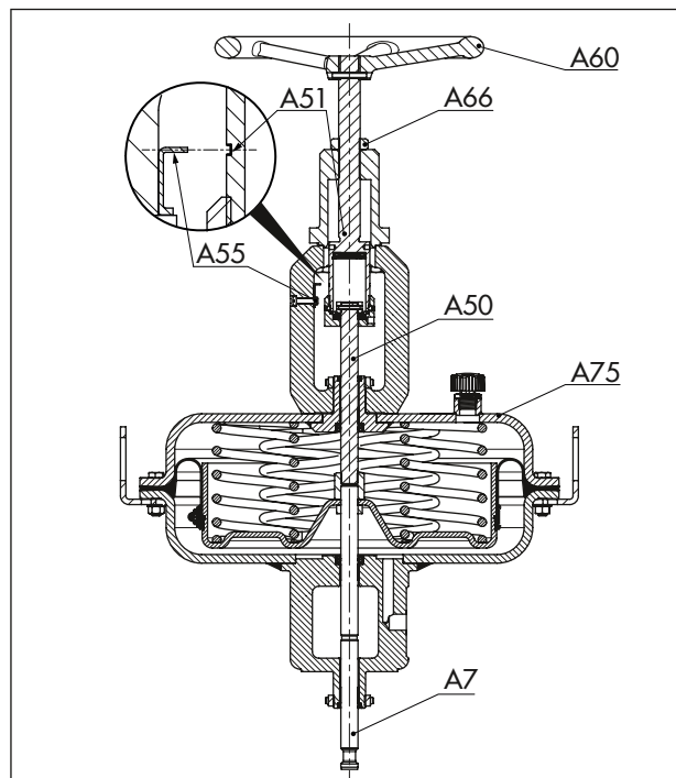
Bild 20: Pneumatischer Antrieb Typ 3277 mit Handverstellung
