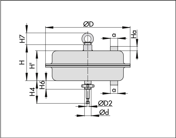
Bild 4: Typ 3271 mit 750v2 cm² Antriebsfläche
