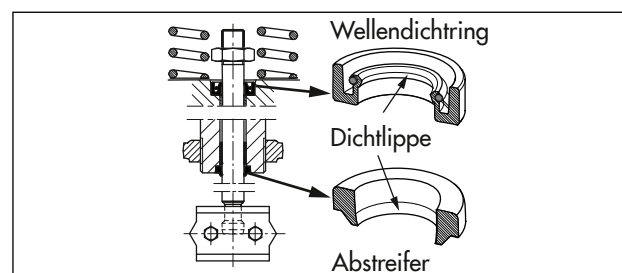
Bild 26: Ausrichtung Wellendichtring und Abstreifer
