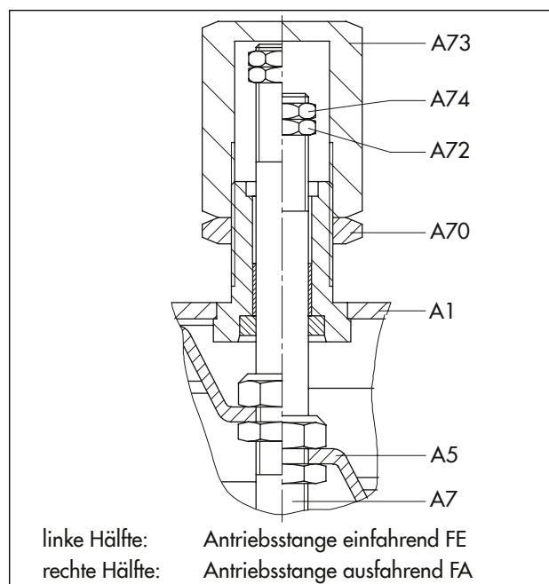
Bild 13: Hubbegrenzung
