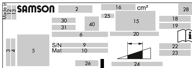
Bild 1: Beschriftungspositionen des Typenschildes am Antrieb Typ 3271/3277 für alle Antriebsflächen >120 cm² oder Typ 3372 mit 350 cm² Antriebsfläche
