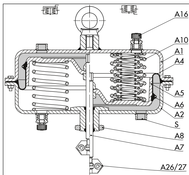
Bild 2: Pneumatischer Antrieb Typ 3271, Beispieldarstellung mit 1400-60 \text{cm}^2 Antriebsfläche
