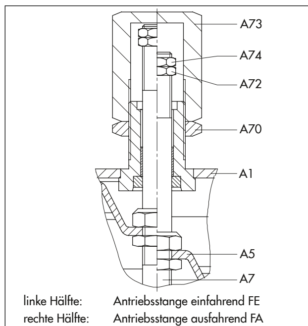
Bild 11: Hubbegrenzung
