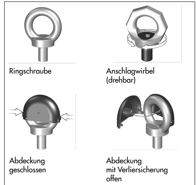
Bild 5: Verliersicherung an Ringschraube/Anschlagwirbel
