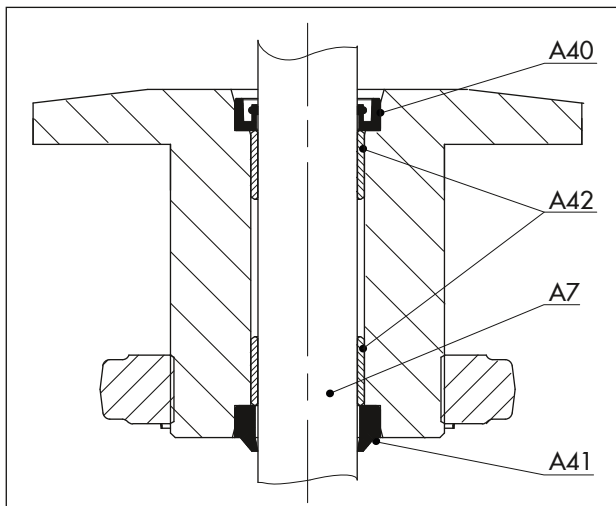
Bild 15: Typ 3271 Antriebsstangendichtung
