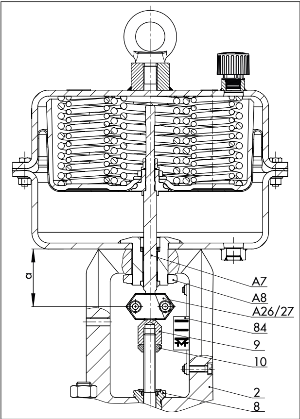
Bild 8: Pneumatischer Antrieb Typ 3271 an Hubventil angebaut
