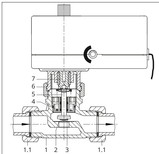
Fig. 3: Type 3222 N/5857 · Type 3222 N/TROVIS 5757-3 · Type 3222 N/TROVIS 5757-7
