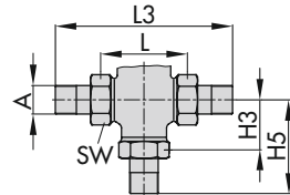
Ausführung mit Außengewinde und Anschraubenden
