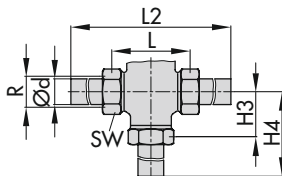
Ausführung mit Außengewinde und Anschweißen
