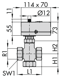
Typ 3226/5857 und Typ 3226/5757-7 nur bis DN 25 Ausführung mit Innengewinde
