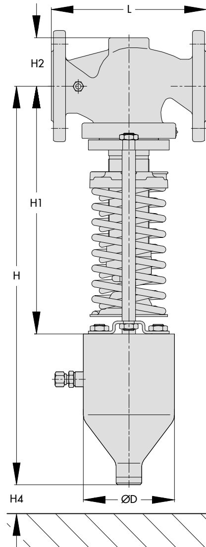
Typ 41-23 mit Balgantrieb
