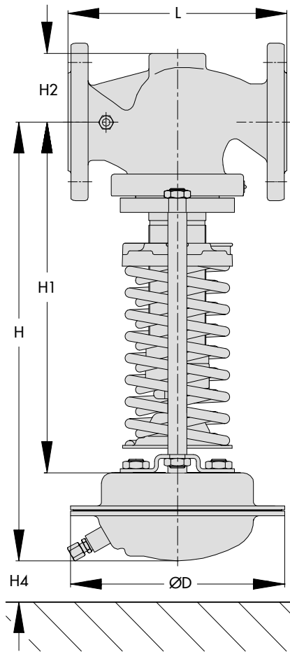
Typ 41-23 mit Membranantrieb
