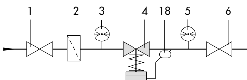
Bild 10: Universal-Druckminderer Typ 41-23, schematisches Einbaubeispiel
