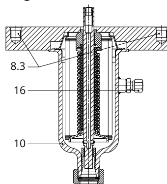
Balgantrieb für DN 65 bis 100
