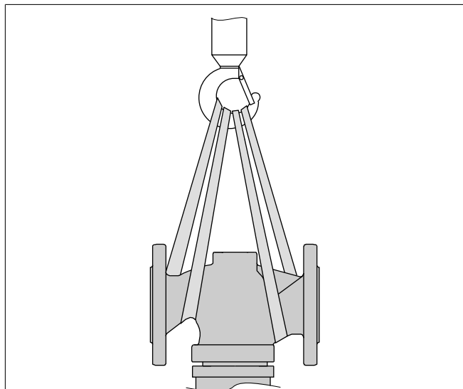
Bild 8: Hebepunkte am Regler, schematische Darstellung
