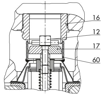
Ausführung mit Strömungsteiler
