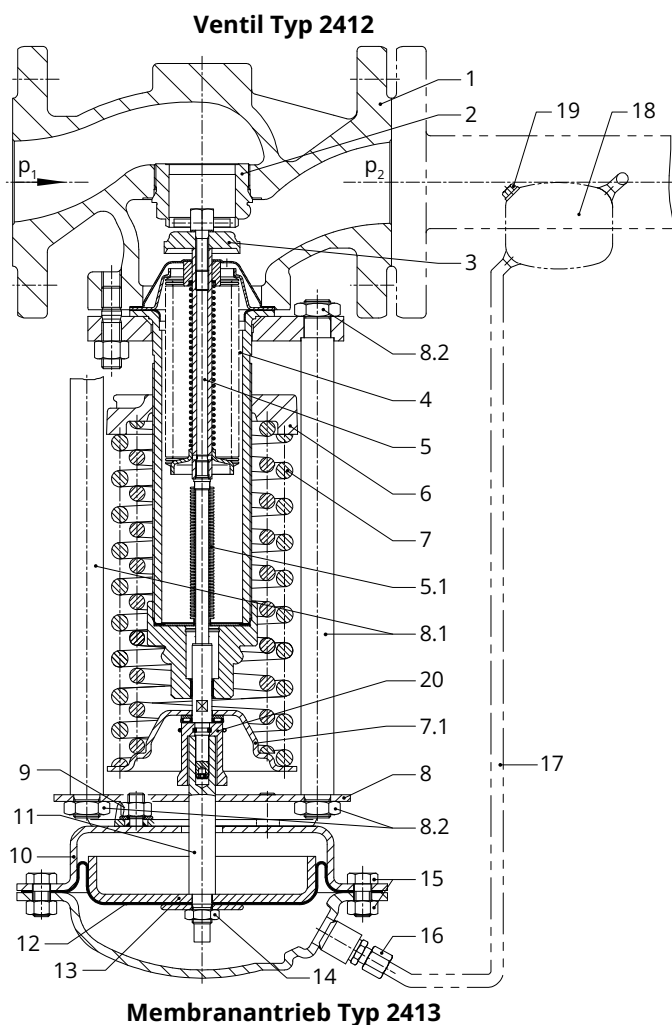
Bild 4: Aufbau und Wirkungsweise, Reglerdarstellung DN 32 bis 100 mit Entlastungsbalg
