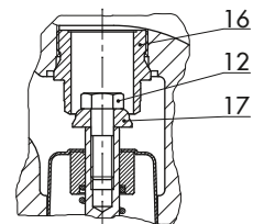
Standardausführung DN 15 bis 25
