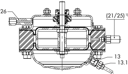
Bild 6: Anschlüsse Membranantrieb Typ 2413
