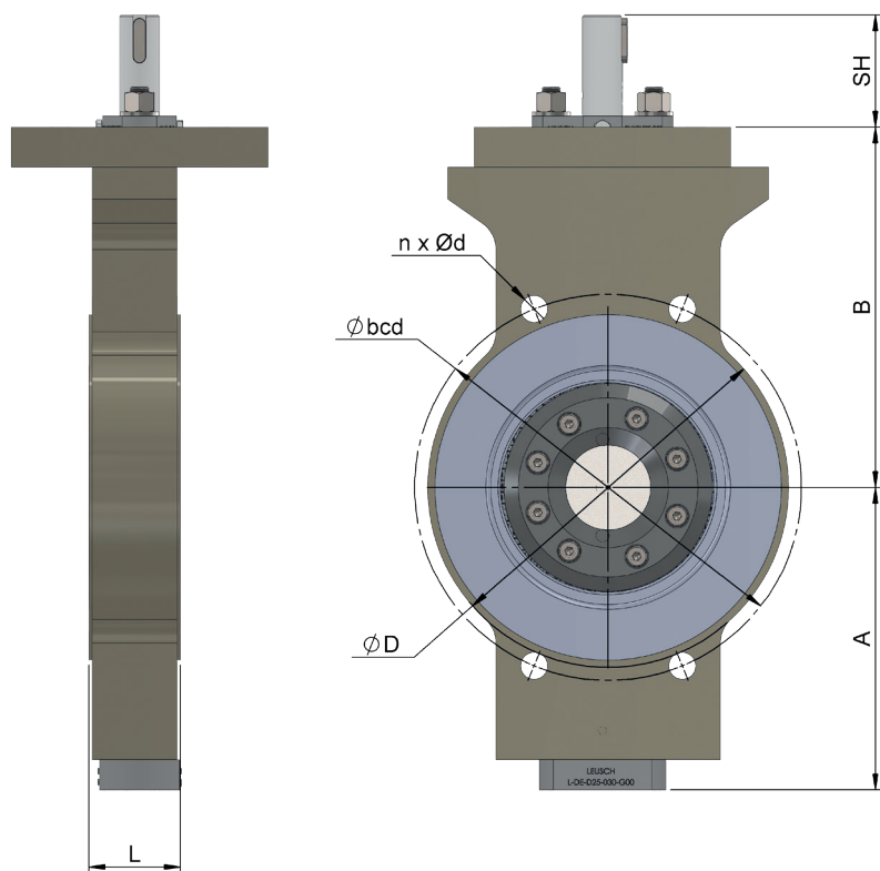
Bild 6: Regel- und Absperrklappe in Zwischenflansch-Design
