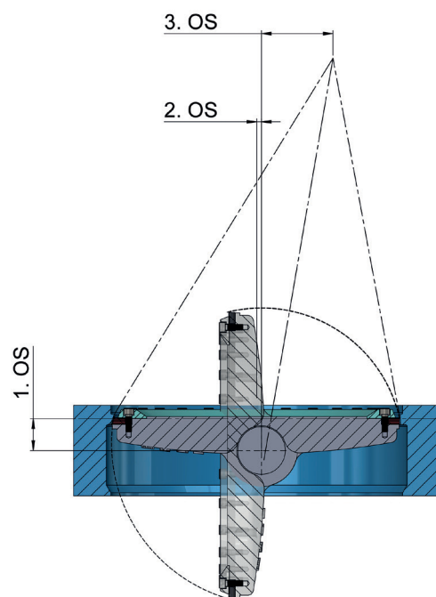
Bild 3: Dreifach-Exzentrizität
