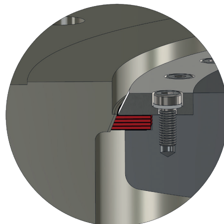
Bild 4: Sitz-Ausführung
