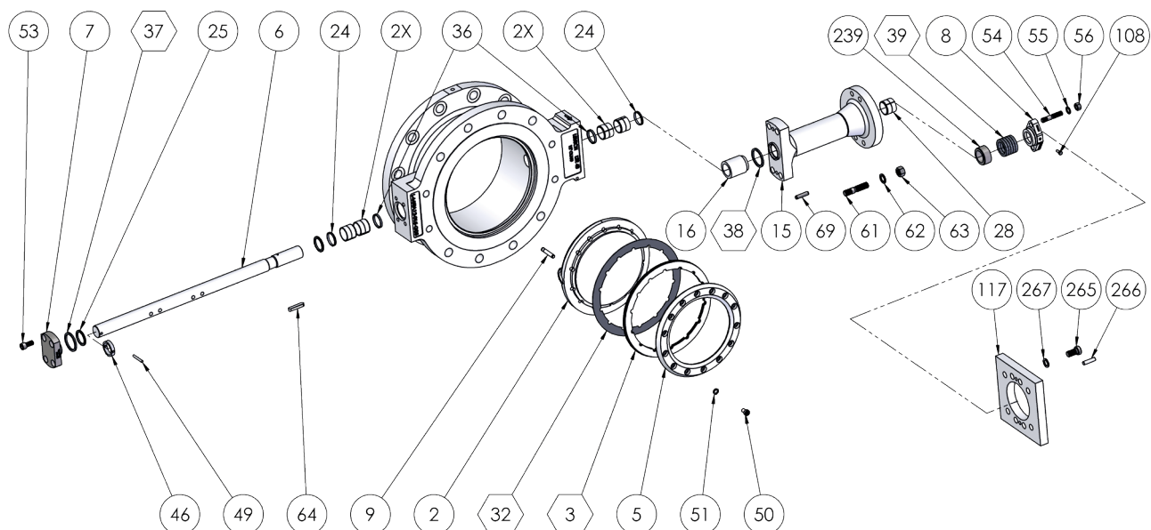
Bild 10: Explosionszeichnung der Regel- und Absperrklappe
