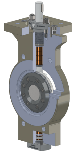
Bild 2: Aufbau der Regel- und Absperrklappe BR 14t - LTR 43
