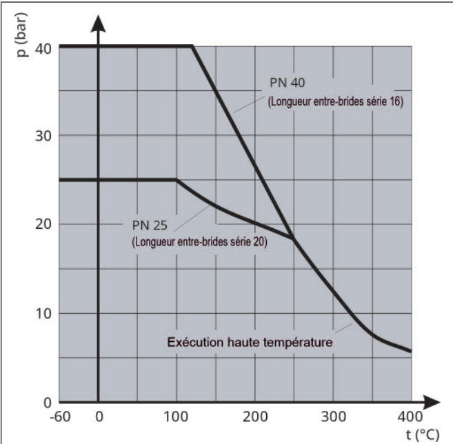
Figure 10: Diagramme pression-température, vanne papillon étanchéité métallique
