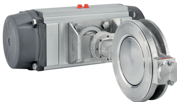
Figure 1: Vanne papillon BR 14b avec servomoteur rotatif BR 31a
