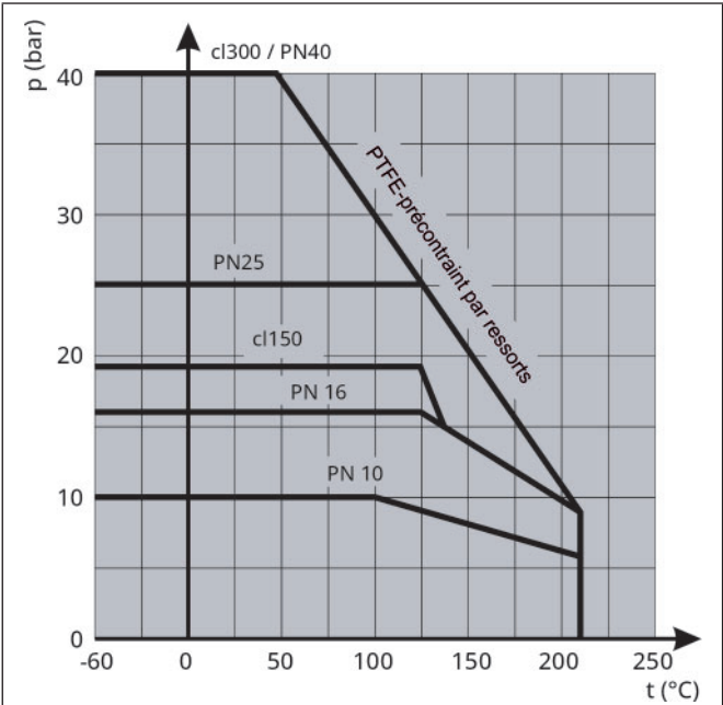
Figure 9: Diagramme pression-température, vanne papillon étanchéité souple
