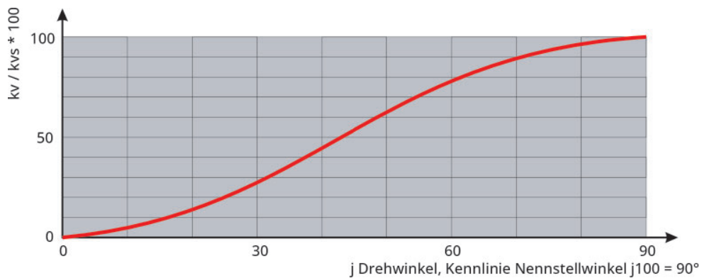
Bild 8: Kennliniendiagramm
